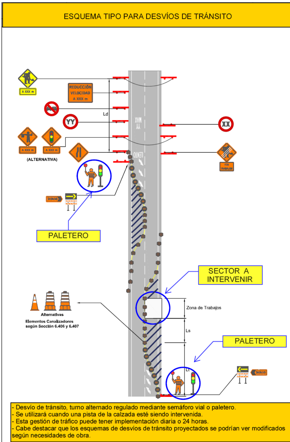
Figura 2: Desvío tipo a realizar en calle Las Romazas (Ruta F-306).
